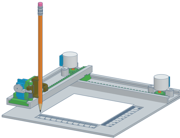
1.1 - Perspectiva
