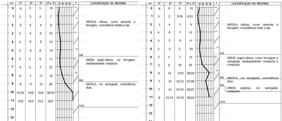
Figura 6: Perfil de sondagem típico da região da Avenida Pierre Chalita, respectivamente SP1 e SP2 Fonte: Empresa X, 2006
