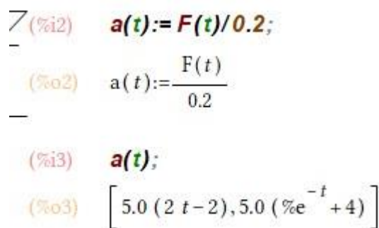
Figura 52 – Encontrando a aceleração em função da força vetorial no WxMaxima.
