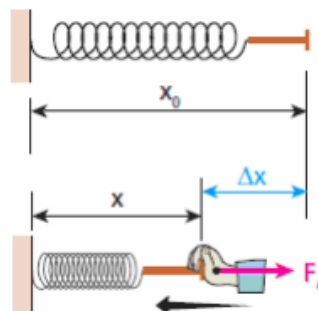
Figura 47 - Alongamento da mola na horizontal.
