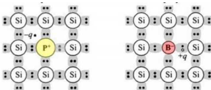
Figura 2.7 (a) Dopagem tipo P do cristal de Si com elemento da família IIIA (Boro). (b) Dopagem tipo N do cristal de Si com elemento da família VA (Fósforo).
