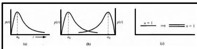
Figura 2.4 (a) Densidade de probabilidade de um átomo isolado. (b) Sobreposição das duas funções de densidade de probabilidade dos átomos adjacentes. (c) Formação da banda de energia para o estado n = 1
