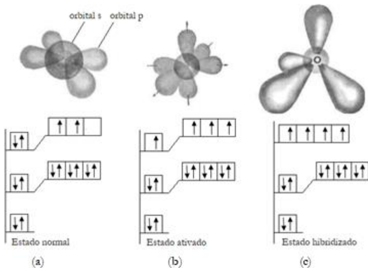
Figura 2.2 Hibridização do Si no processo de formação da molécula.
