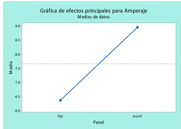
Figura 11. Gráfico de efectos principales de Amperaje (Elaboración propia)
