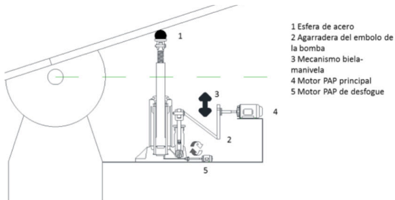
Figura 2. Mecanismo de elevación y cambio de ángulo (Elaboración propia)
