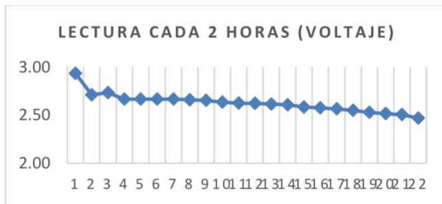
Figura 5. Consumo de corriente (Elaboración propia)
