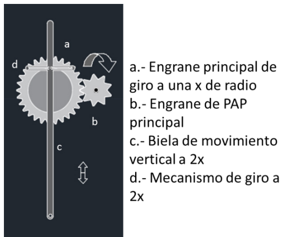
Figura 3. Mecanismo de movimiento vertical (Elaboración propia)
