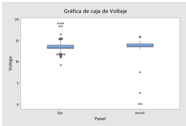
Figura 14. Gráfico de caja de Voltaje (Elaboración propia)
