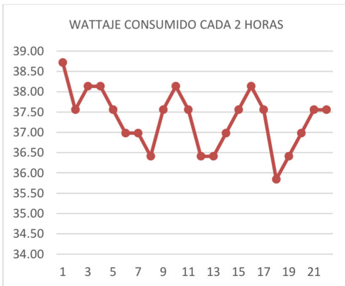
Figura 10. Potencia disipada (Elaboración propia)
