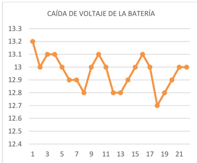
Figura 9. Caída de tensión en 22 horas (Elaboración propia)
