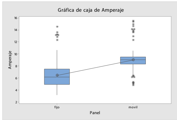
Figura 13. Gráfico de caja de Amperaje (Elaboración propia)
