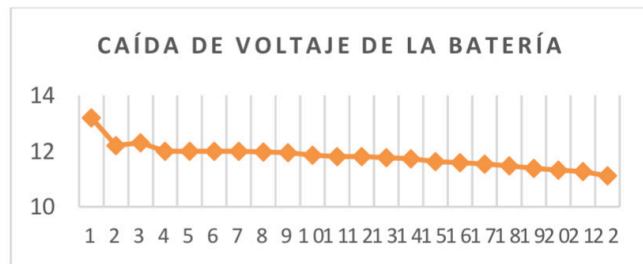
Figura 6. Caída de tensión en 22 horas (Elaboración propia)
