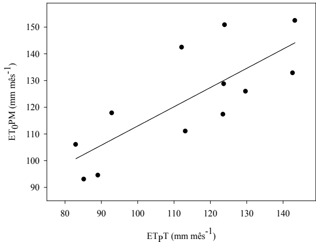
Figura 3 - Análise de regressão linear para Evapotranspiração Potencial pelo método de Thornthwite (ET o T) e Evapotranspiração de Referência, calculada pelo método padrão, Penman-Monteith (FAO56) (ET o PM), do ano de 2019 em Rio Largo, Alagoas.
