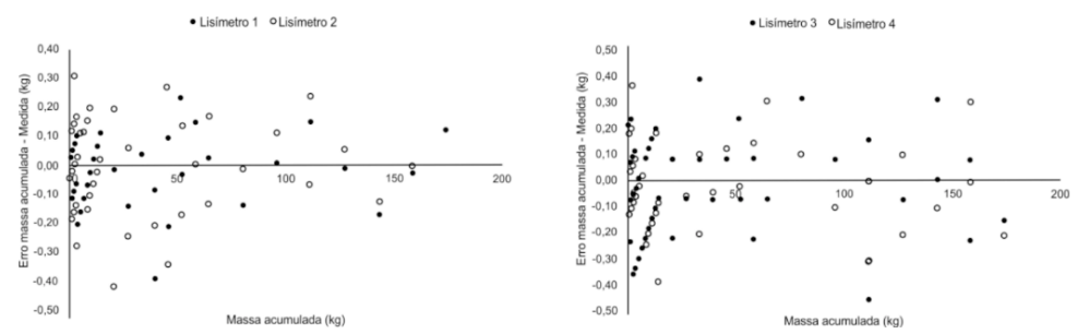
Figura 2. Erros entre a massa acumulada e a massa determinada durante a calibração dos lisímetros.
