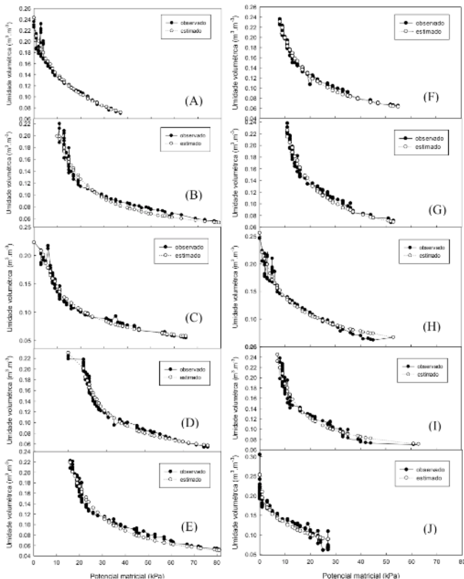
Figura 1. Curva de retenção de água para os substratos preparados com 100% substrato (A), 100% solo (B), 90% solo + 10% substrato (C); 80% solo + 20% substrato (D); 70% solo+30% substrato (E); 60% solo + 40% de substrato (F); 50% solo + 50% substrato (G); 40% solo + 60% substrato (H); 30% solo+70% substrato (I) e 20% solo+80% substrato (J).
