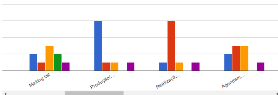
Gráfico 17 – Especifique com que frequência você desempenha as funções abaixo na assessoria de imprensa, parte 2
