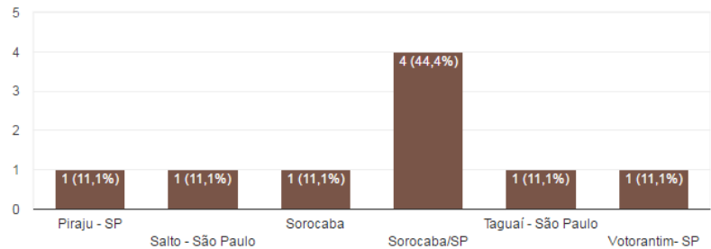
Gráfico 3 – Cidade e estado onde nasceu Elaborado pela autora.
