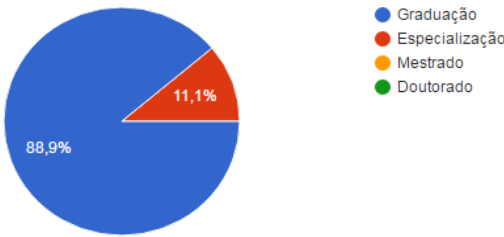
Gráfico 7 – Titulação Elaborado pela autora.
