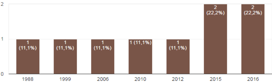
Gráfico 8 – Ano de conclusão da graduação Elaborado pela autora.
