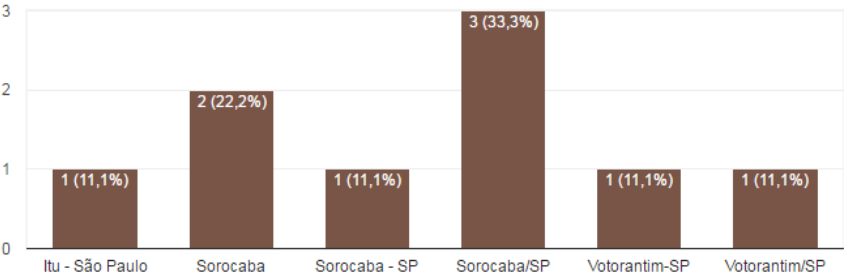
Gráfico 4 – Cidade e estado onde reside atualmente
