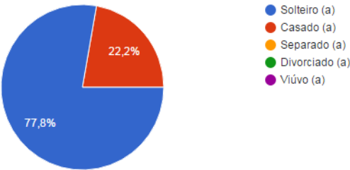
Gráfico 2 – Estado civil Elaborado pela autora.
