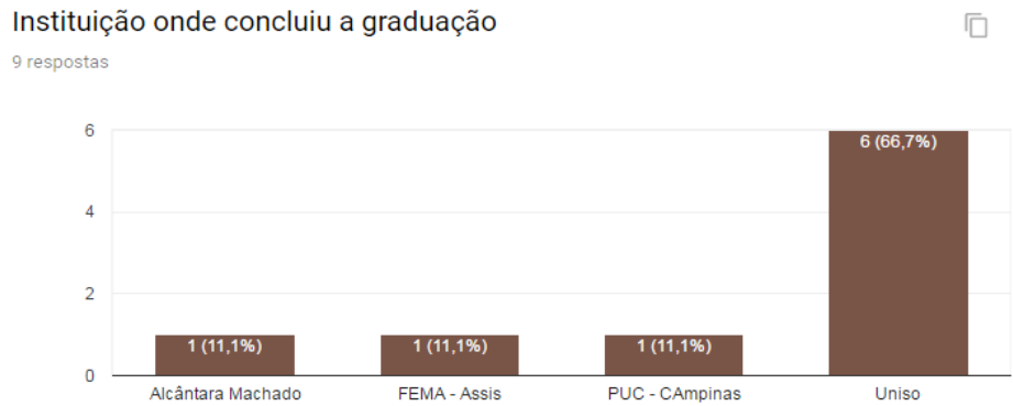
Gráfico 9 – Instituição onde concluiu a graduação Elaborado pela autora.
