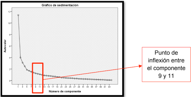
Figura 2. Análisis de factores confirmatorio: Gráfico de sedimentación en SPSS v24.
