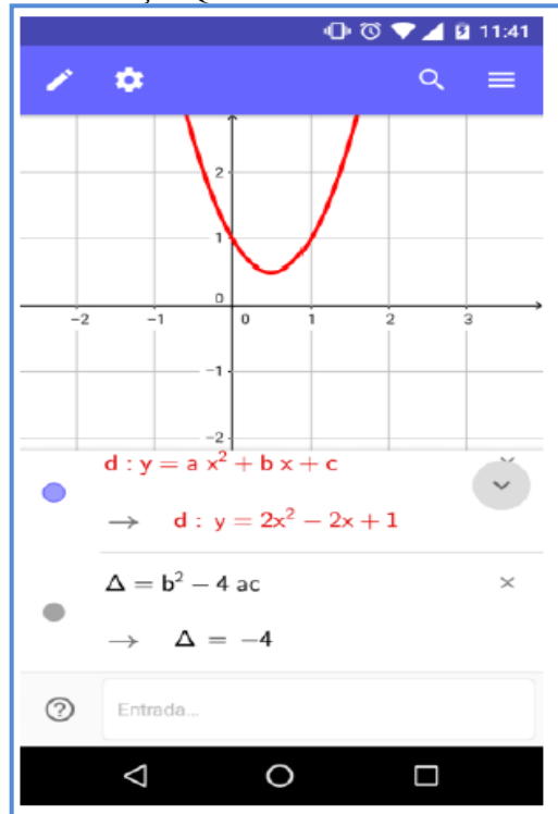
FIGURA 15: Função Quadrática com discriminante negativo.
