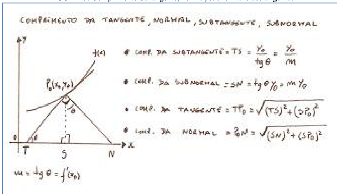
FIGURA 7: Comprimento da tangente, normal, subnormal e subtangente.
