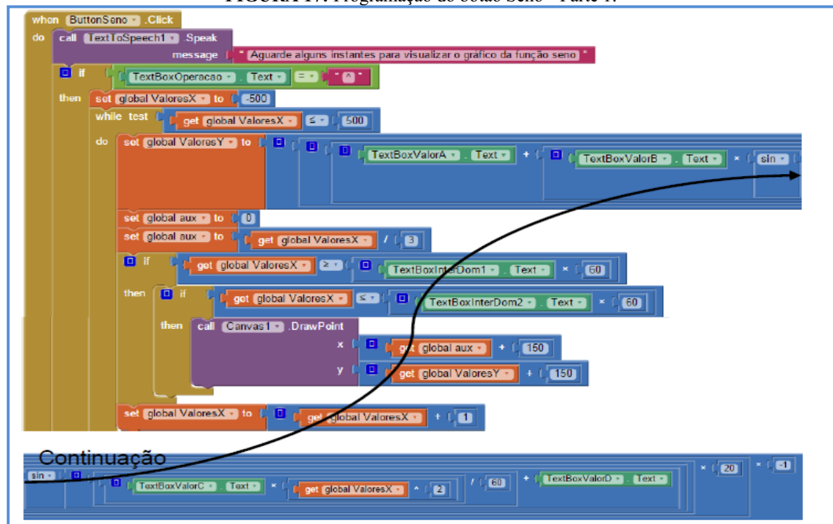
FIGURA 17: Programação do botão Seno - Parte 1.
