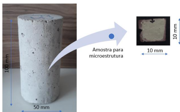
Figura 2. Extração de amostra do corpo de prova para análise de microestrutura.
