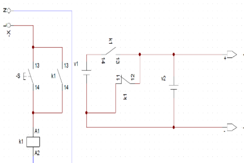
Figura 8. Circuito de comando da associação das baterias.
