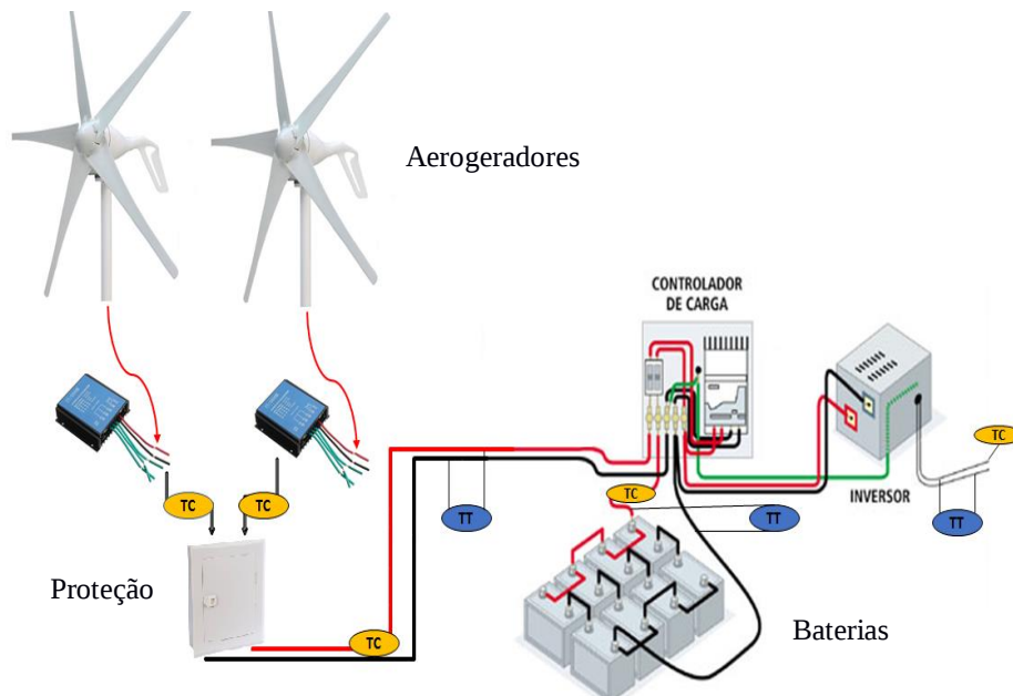
Legenda: TT –transdutor de tensão; TC – transdutor de corrente. Figura 7. Descrição do sistema de micro geração eólica.
