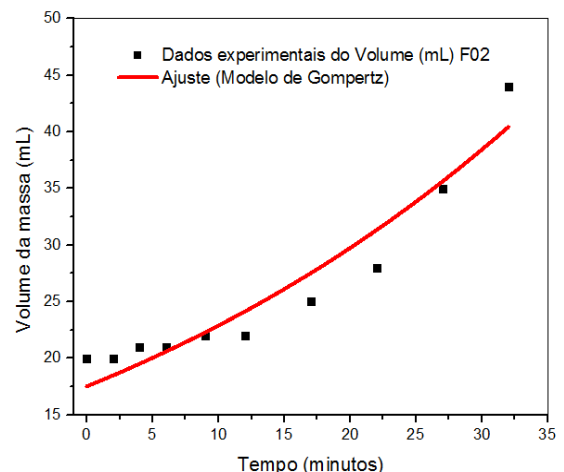
Figura 12. Dados experimentais do volume da fermentação pelo tempo da F2 (goma xantana) ajustados pelo modelo de crescimento Gompertz.
