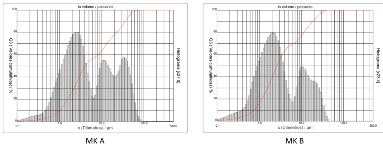
Figura 3. Distribuição granulométrica.
