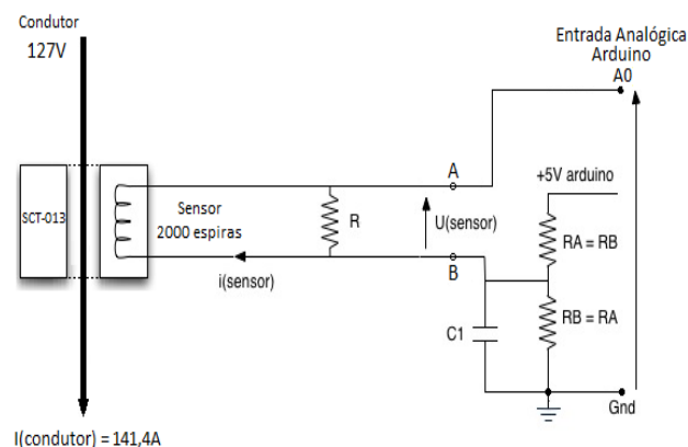
Figura 1. Esquema de ligação do sensor de corrente. C1=10μF, R=330 Ω e RA=RB=10kΩ.
