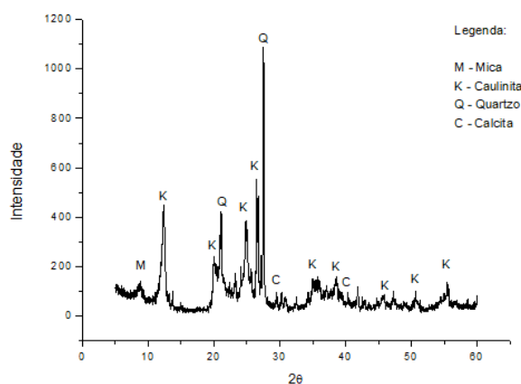
Figura 7. Difração de raios X do solo.
