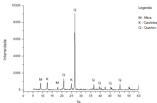
Figura 12. Difração de raios X do resíduo de caulim grosso.
