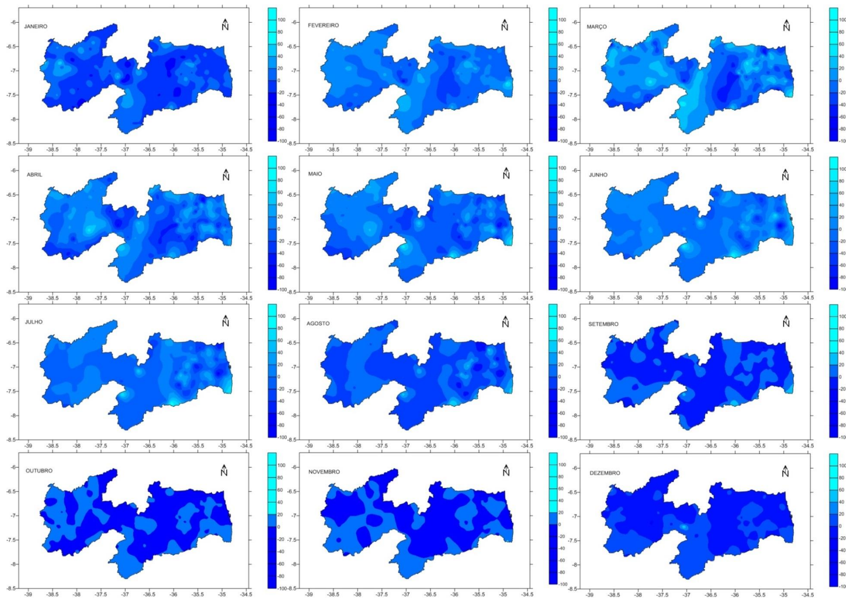
Figura 17. Flutuação mensal da precipitação.
