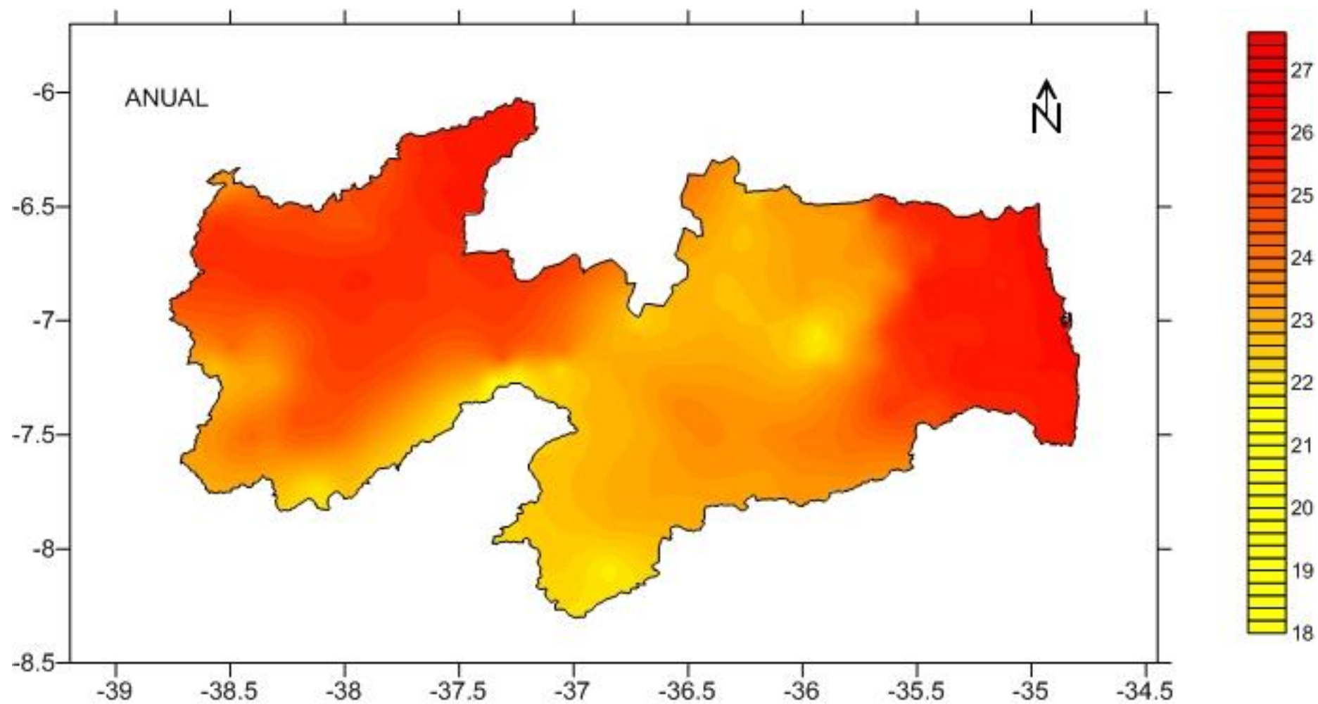
Figura 5. Temperatura média anual (°C).
