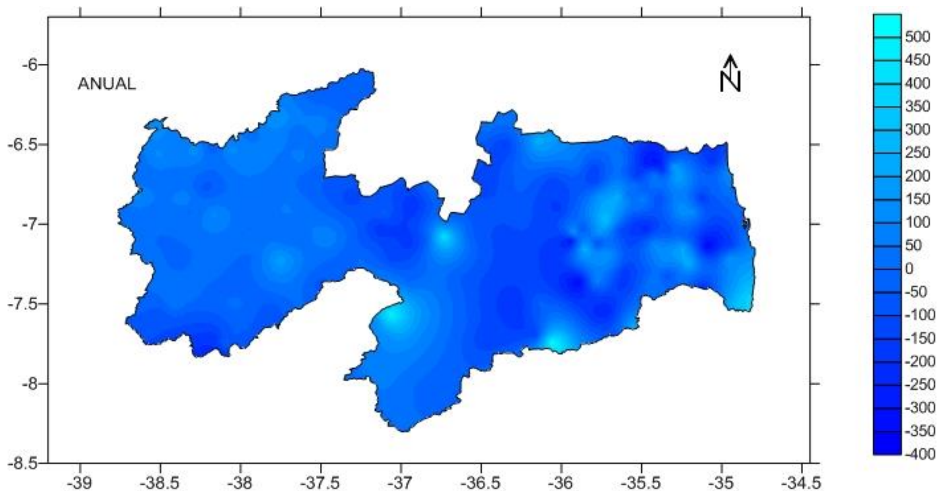
Figura 18. Flutuação anual da precipitação.
