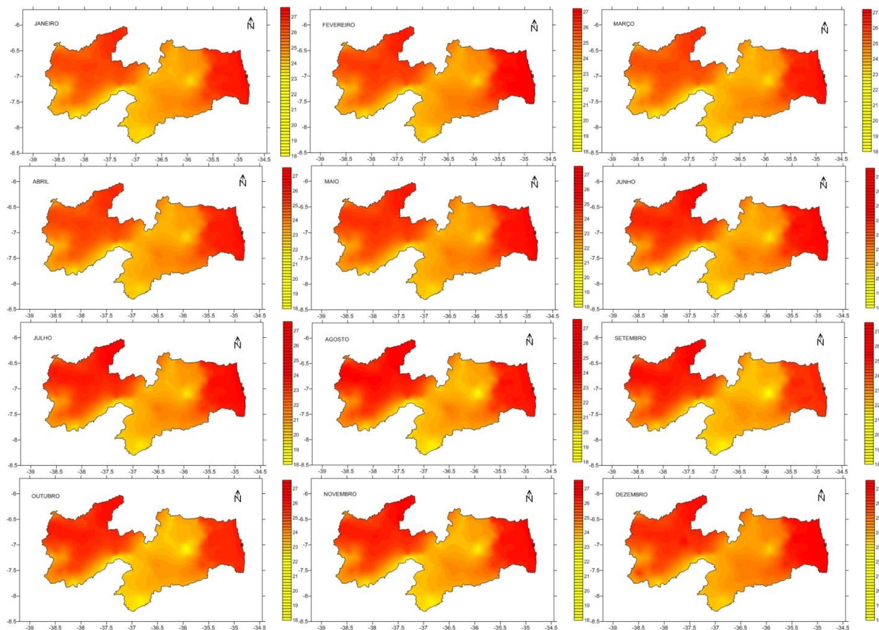
Figura 4. Temperatura média mensal do Estado da Paraíba (°C).
