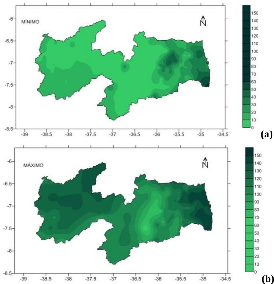
Figura 28. Distribuição mínima (a) e máxima (b) da evaporação no Estado da Paraíba.
