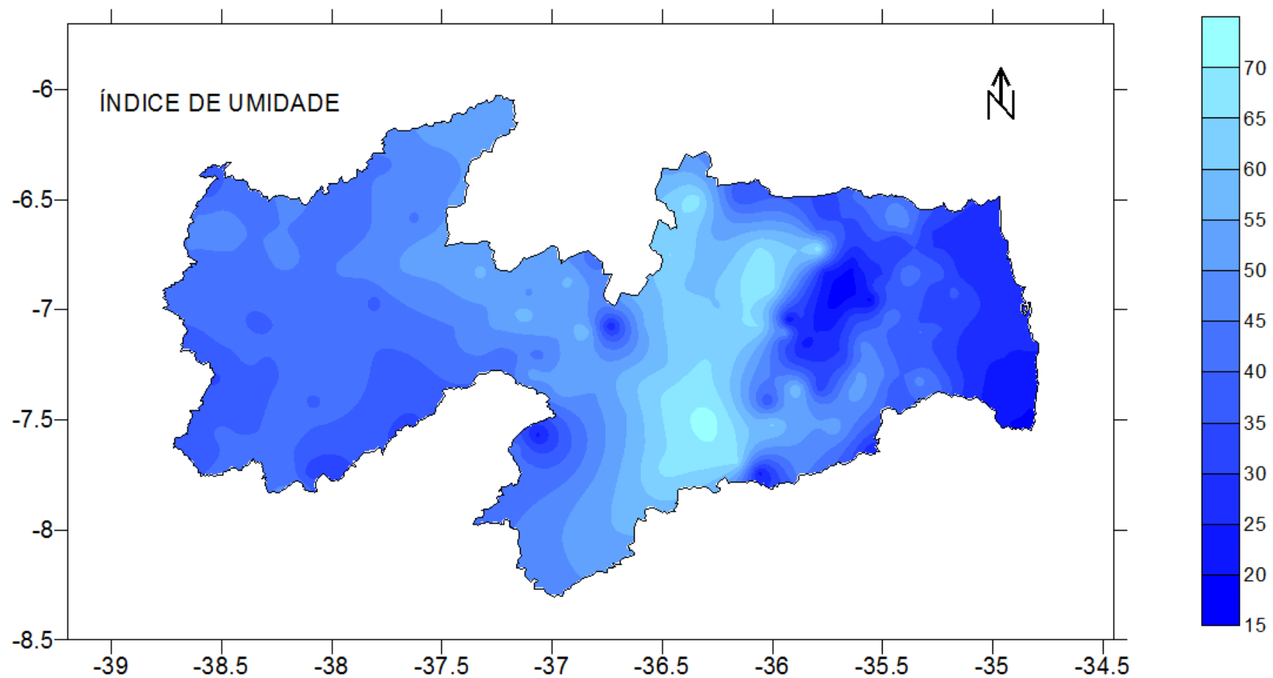
Figura 32. Índice de umidade (iu).
