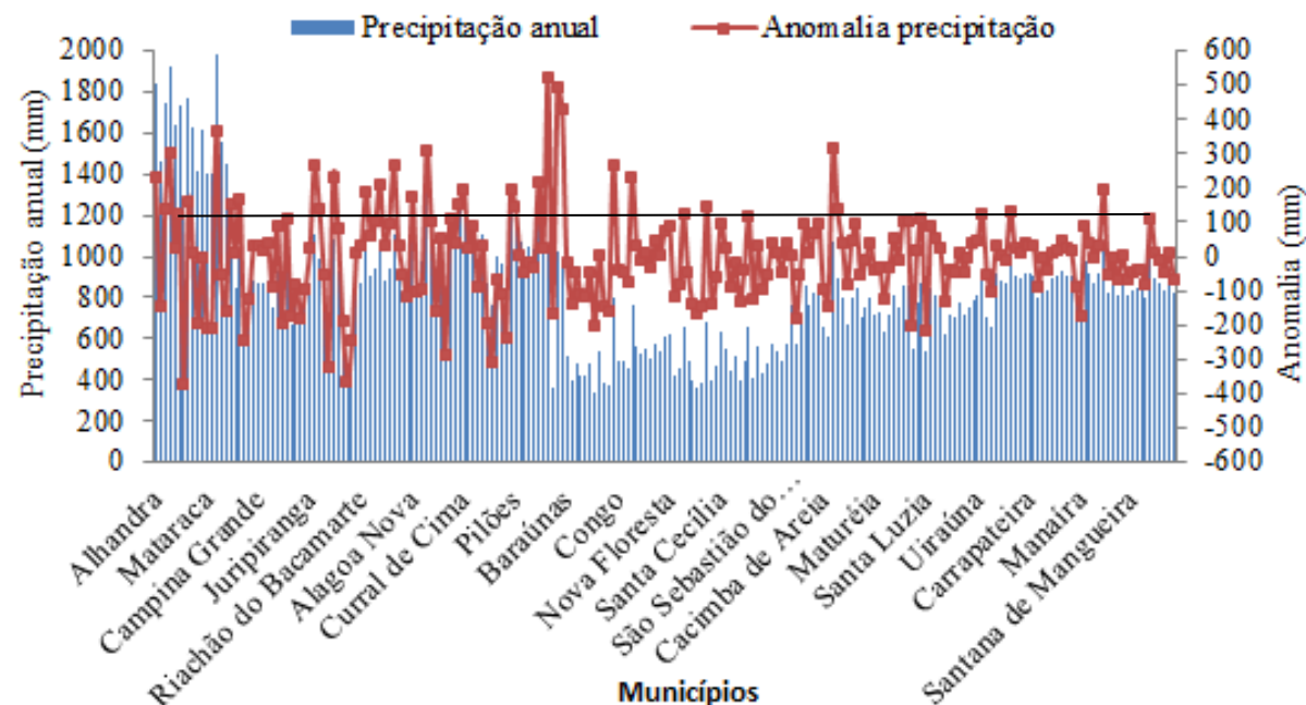
Figura 21. Precipitação anual e anomalia.
