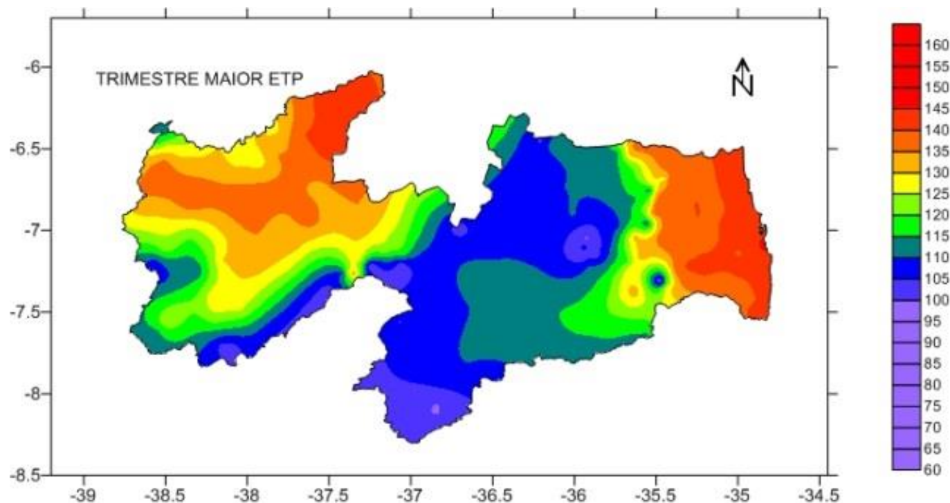
Figura 25. Trimestre de maior ETP.
