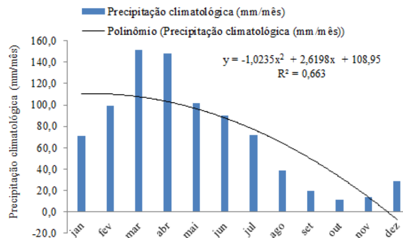
Figura 16. Histograma da média pluviométrica climatológica e tendência polinomial.
