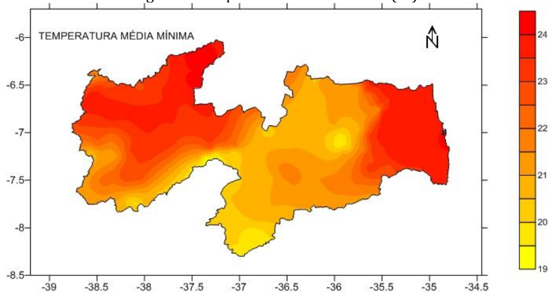
Figura 9. Temperatura média mínima (°C).
