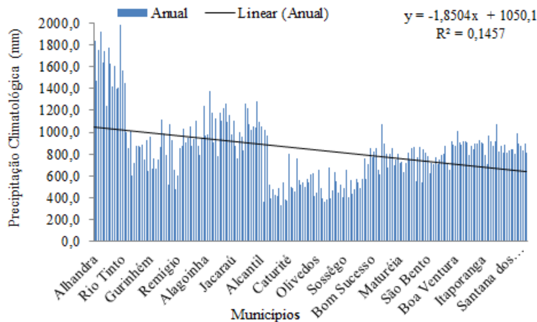
Figura 14. Distribuição espaço-temporal e análise de regressão linear da precipitação anual.
