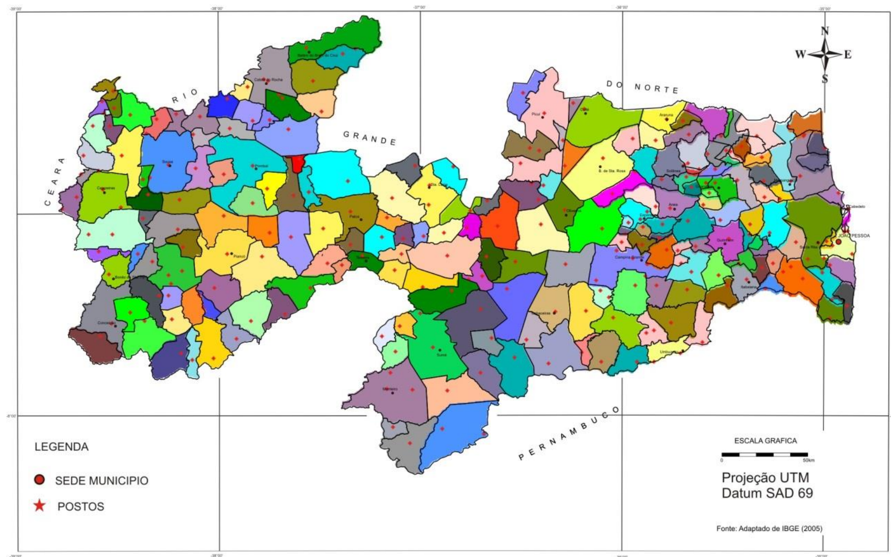
Figura 3. Distribuição espacial dos postos pluviométricos do Estado da Paraíba. Fonte: Adaptado de IBGE (2005).
