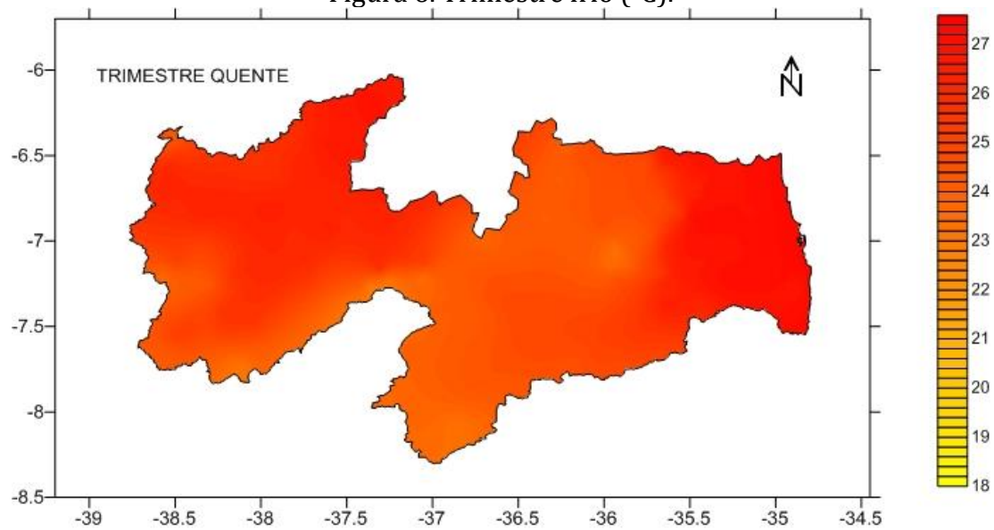
Figura 7. Trimestre quente (°C).
