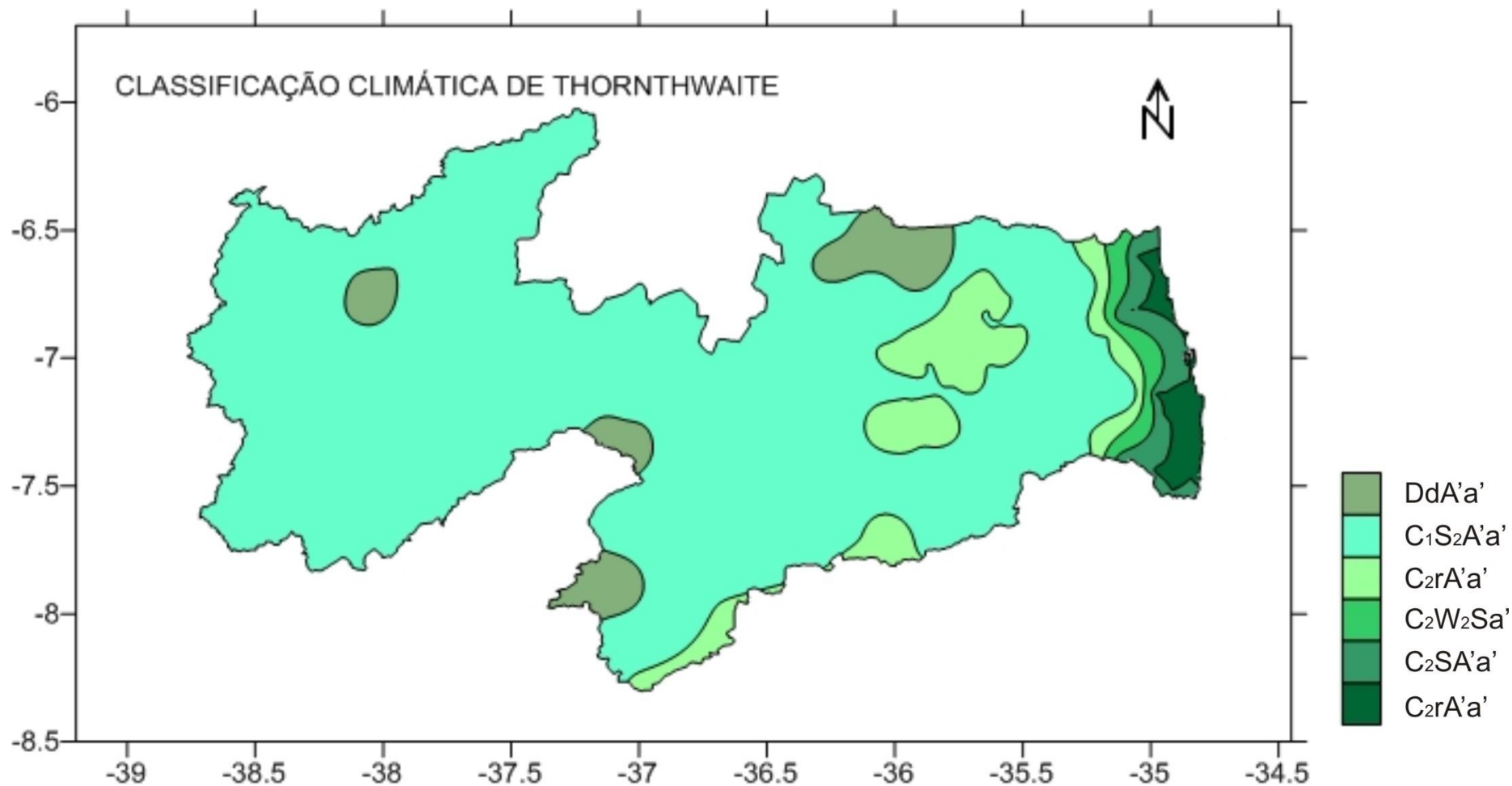
Figura 36. Classificação climática de Thornthwaite normal.
