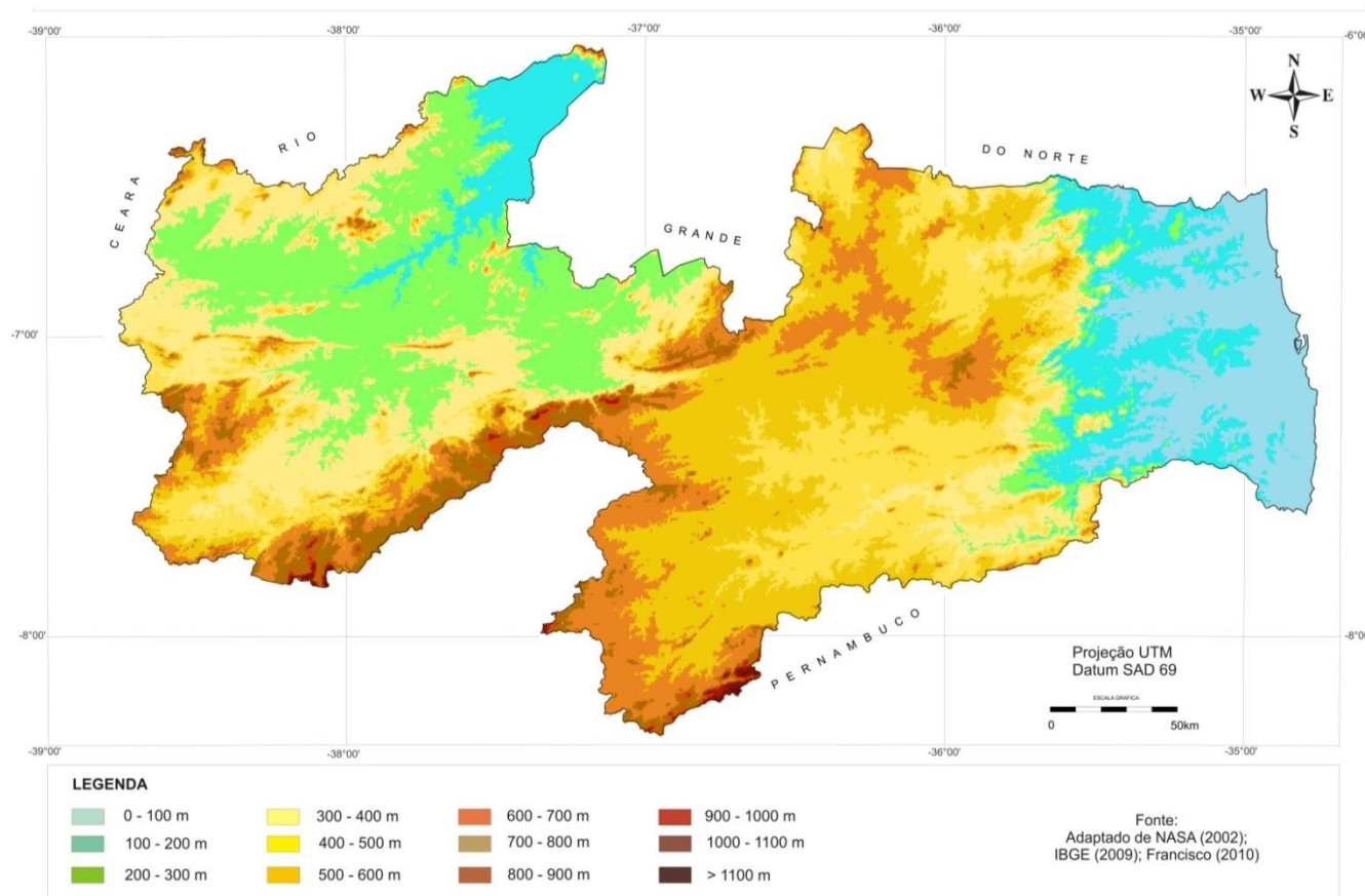
Figura 2. Mapa hipsométrico do Estado da Paraíba. Fonte: Francisco et al. (2014).
