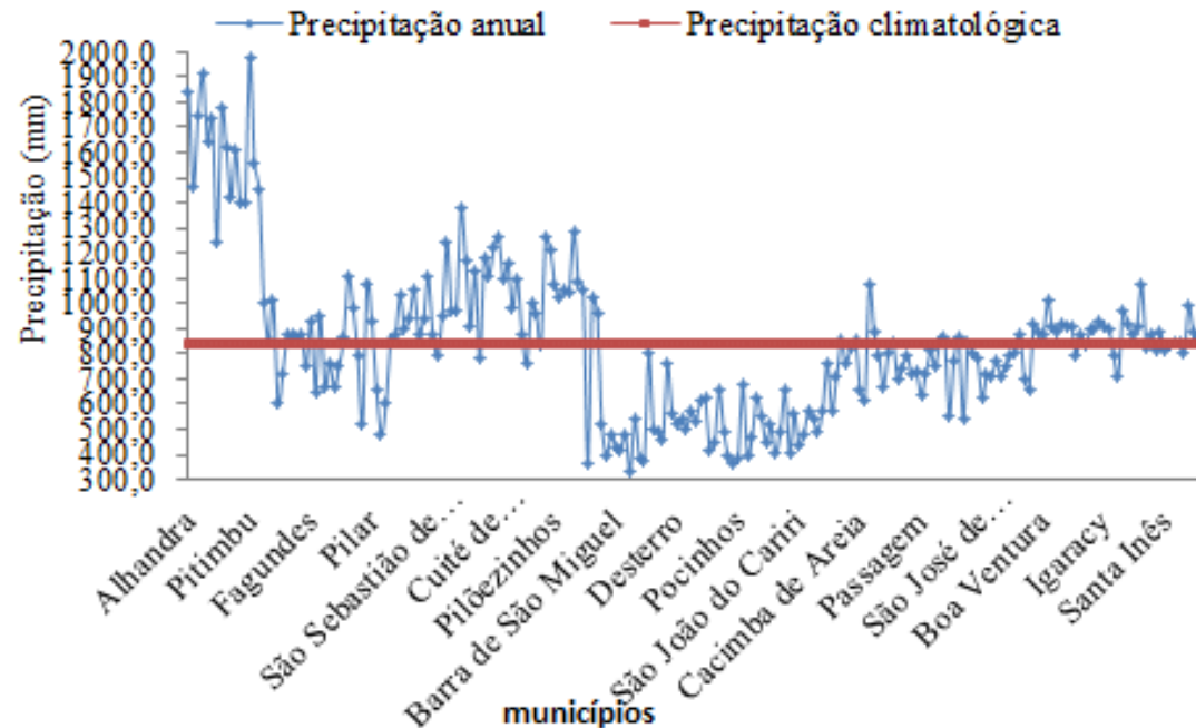
Figura 19. Distribuição temporal da precipitação anual e da média climatológica.
