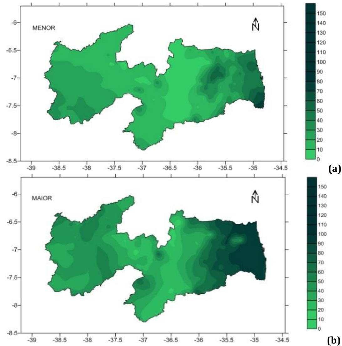
Figura 29. Distribuição do trimestre de menor (a) e maior (b) evaporação no Estado da Paraíba.
