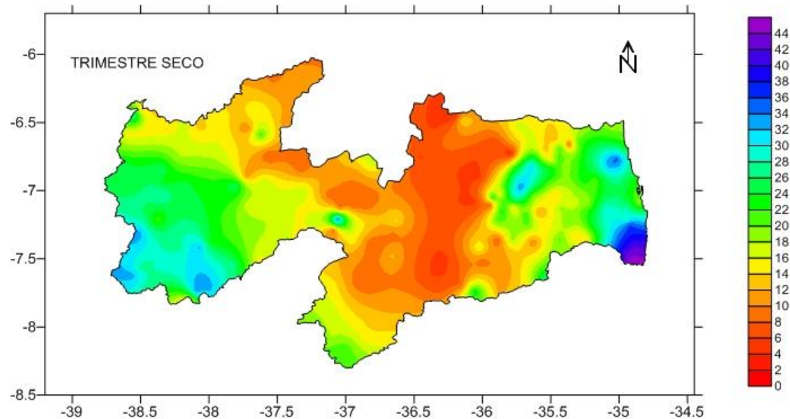
Figura 13. Pluviosidade média do trimestre seco (mm).
