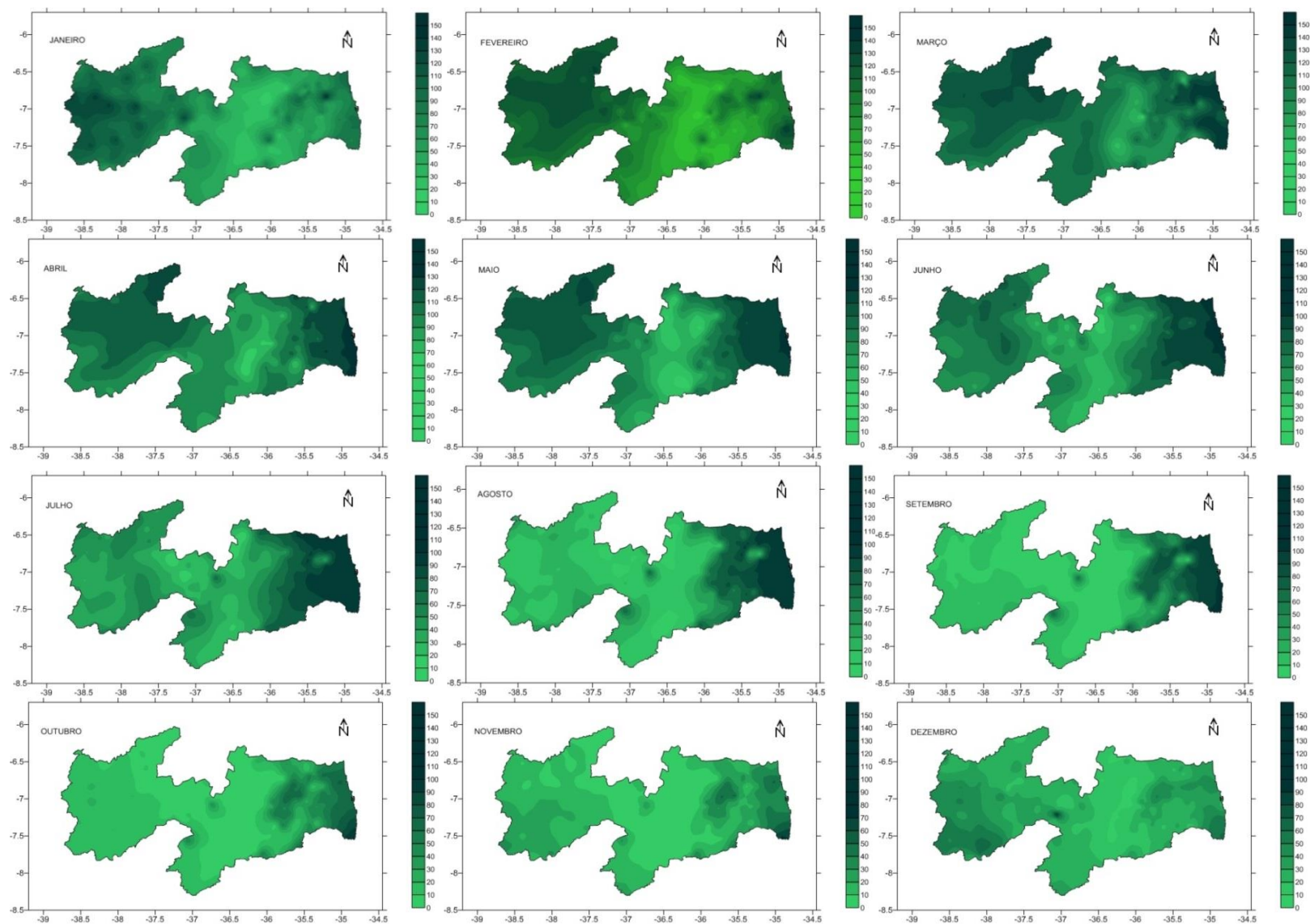
Figura 26. Distribuição mensal da evaporação no Estado da Paraíba.
