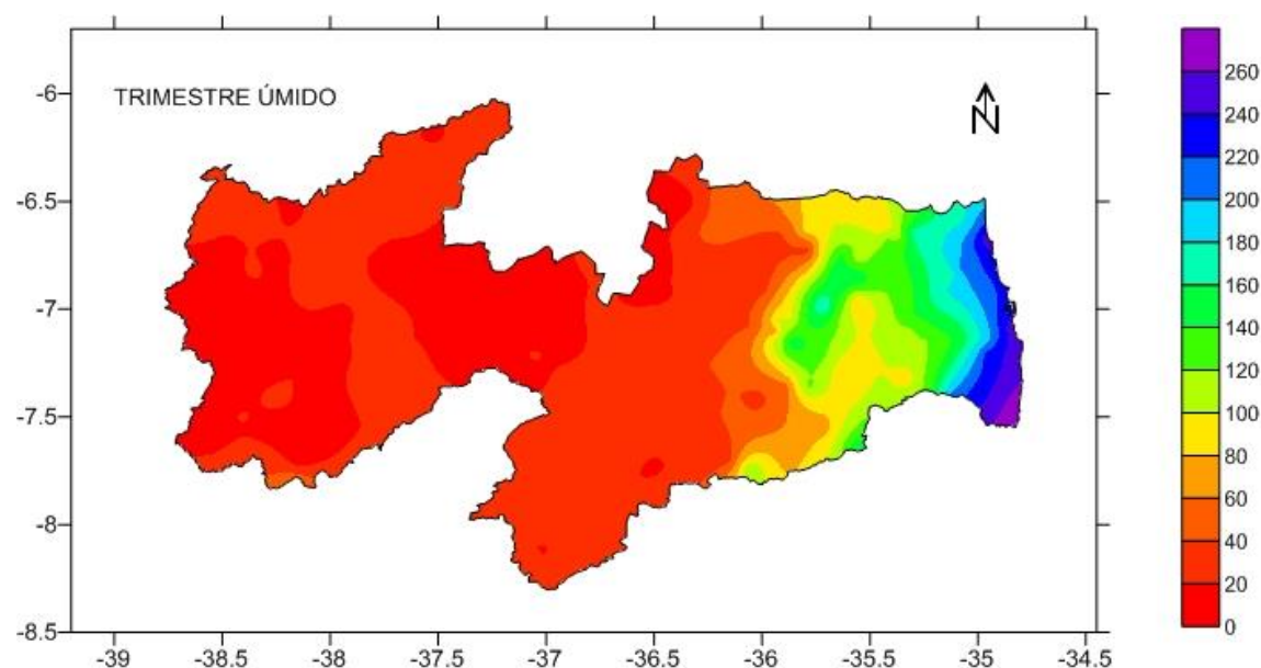
Figura 12. Pluviosidade média do trimestre úmido (mm).
