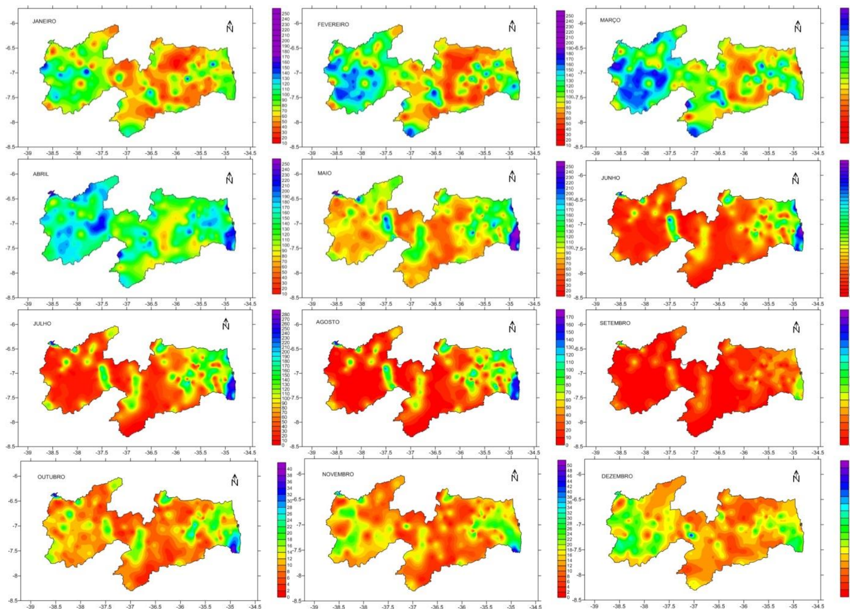
Figura 10. Pluviosidade mensal média (mm).
