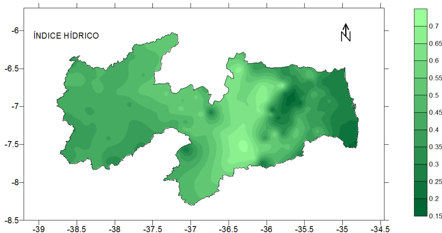
Figura 33. Índice hídrico (ih).
