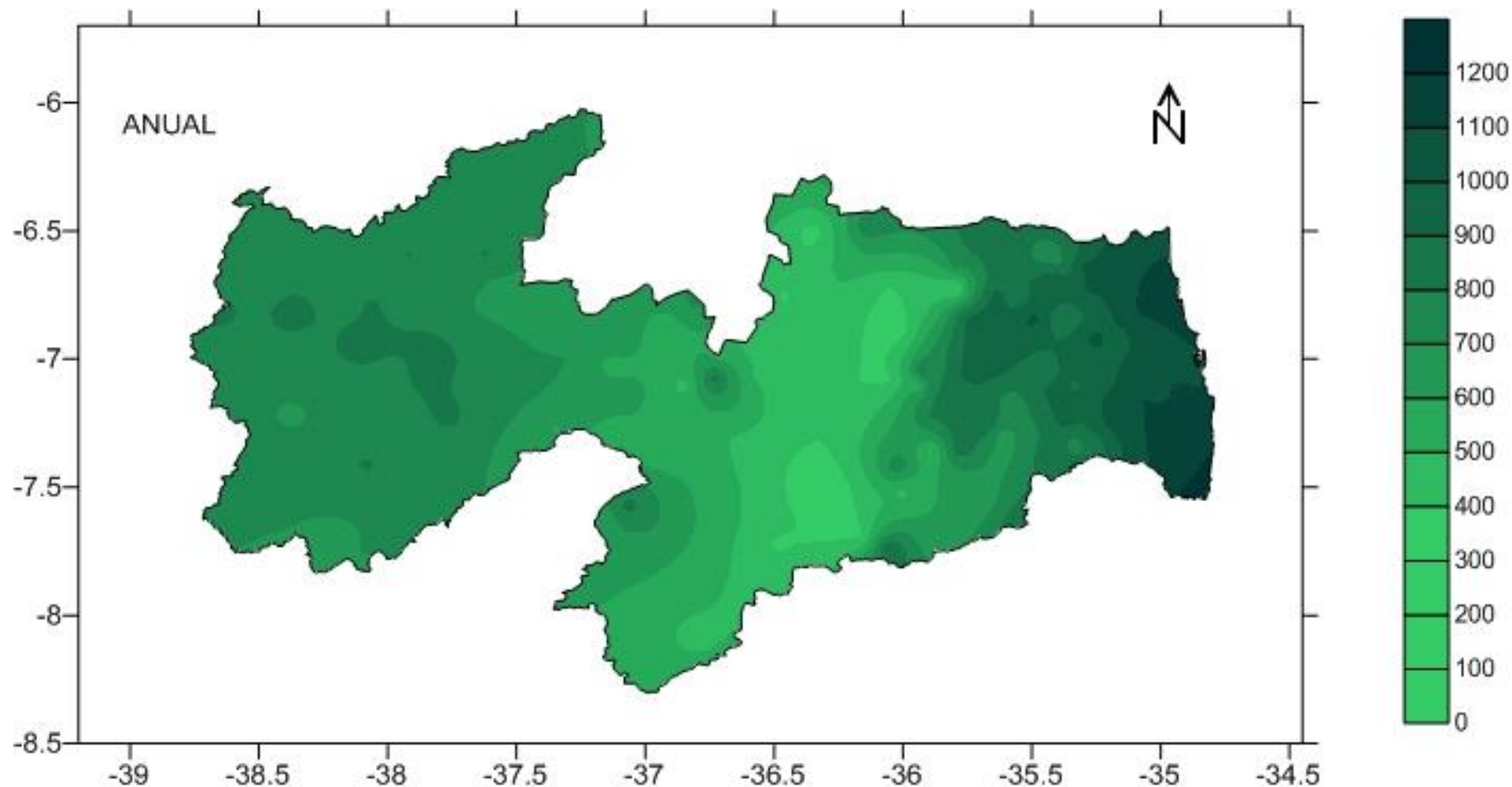
Figura 27. Distribuição anual da evaporação no Estado da Paraíba.
