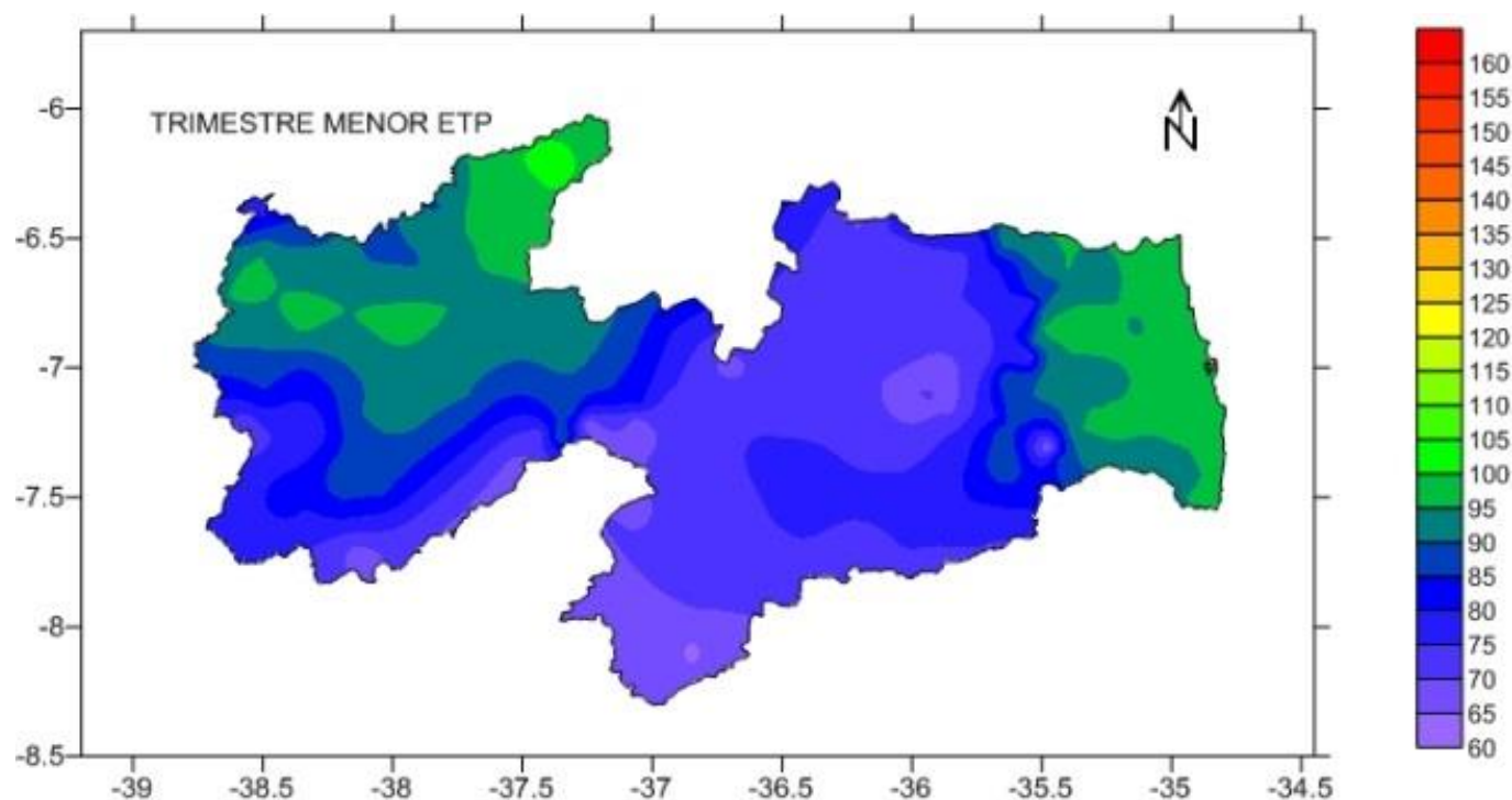
Figura 24. Trimestre de menor ETP.
