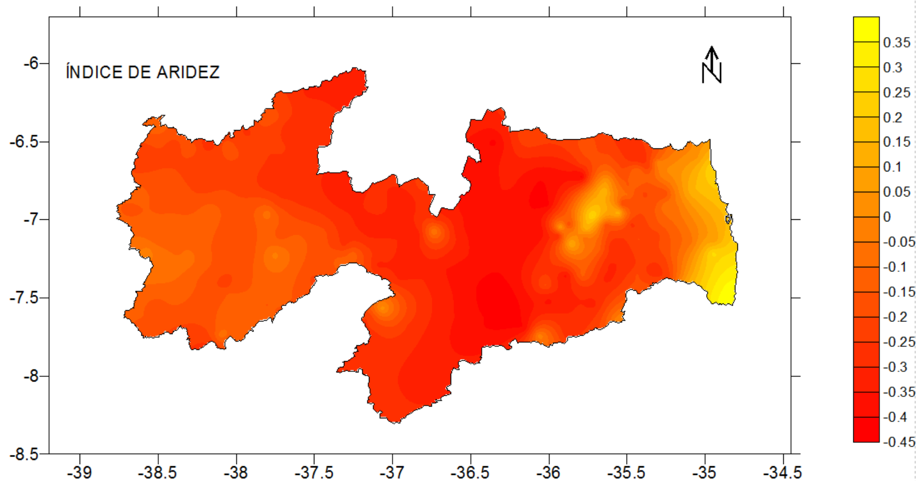
Figura 34. Índice de aridez (ia).
