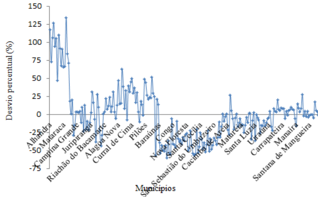
Figura 20. Desvio percentual anual da precipitação em relação à média histórica.
