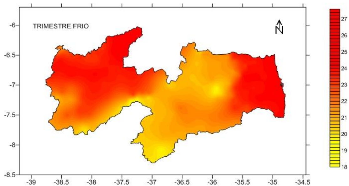
Figura 6. Trimestre frio (°C).
