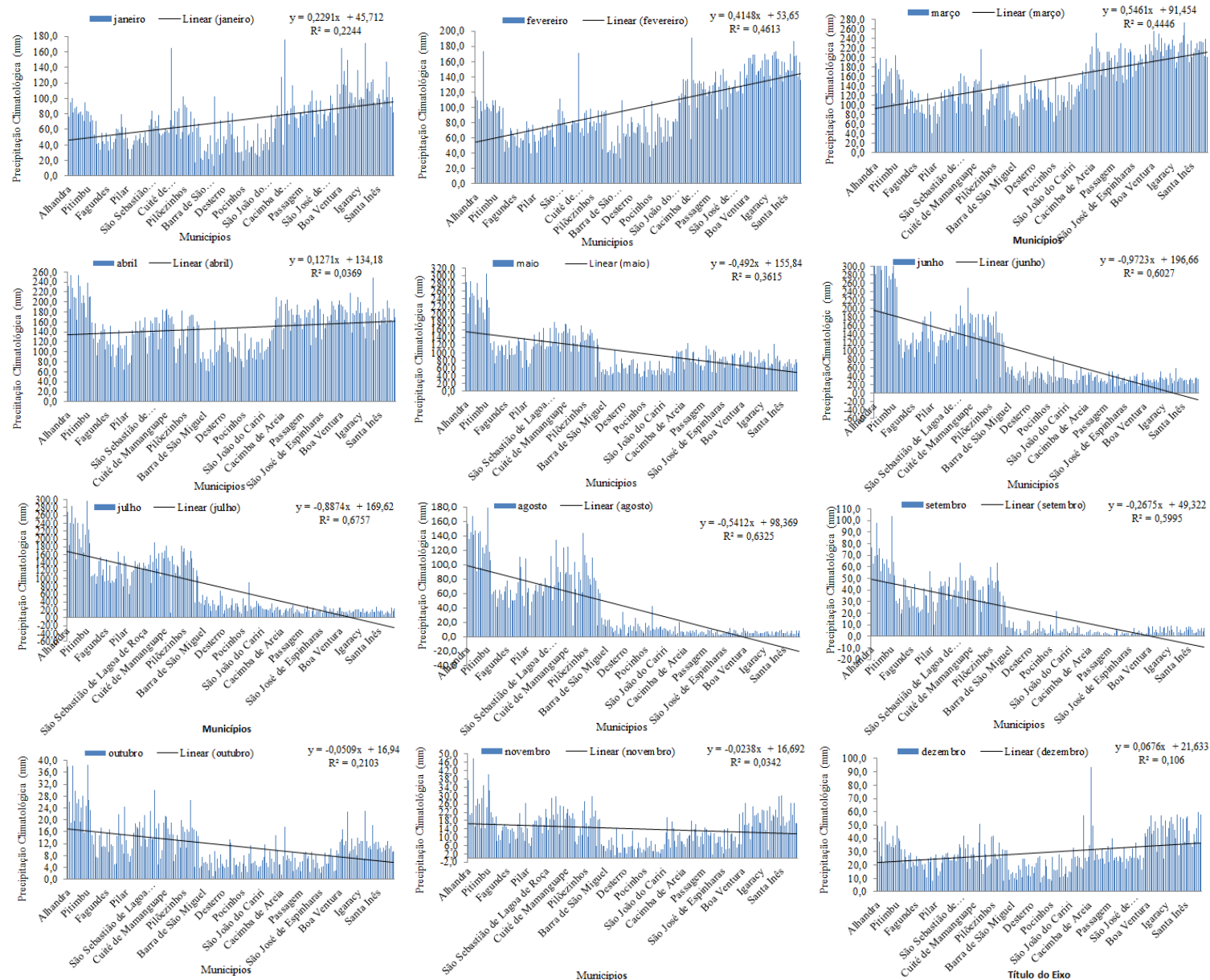
Figura 15. Distribuição espaço-temporal das precipitações pluviais mensais.
