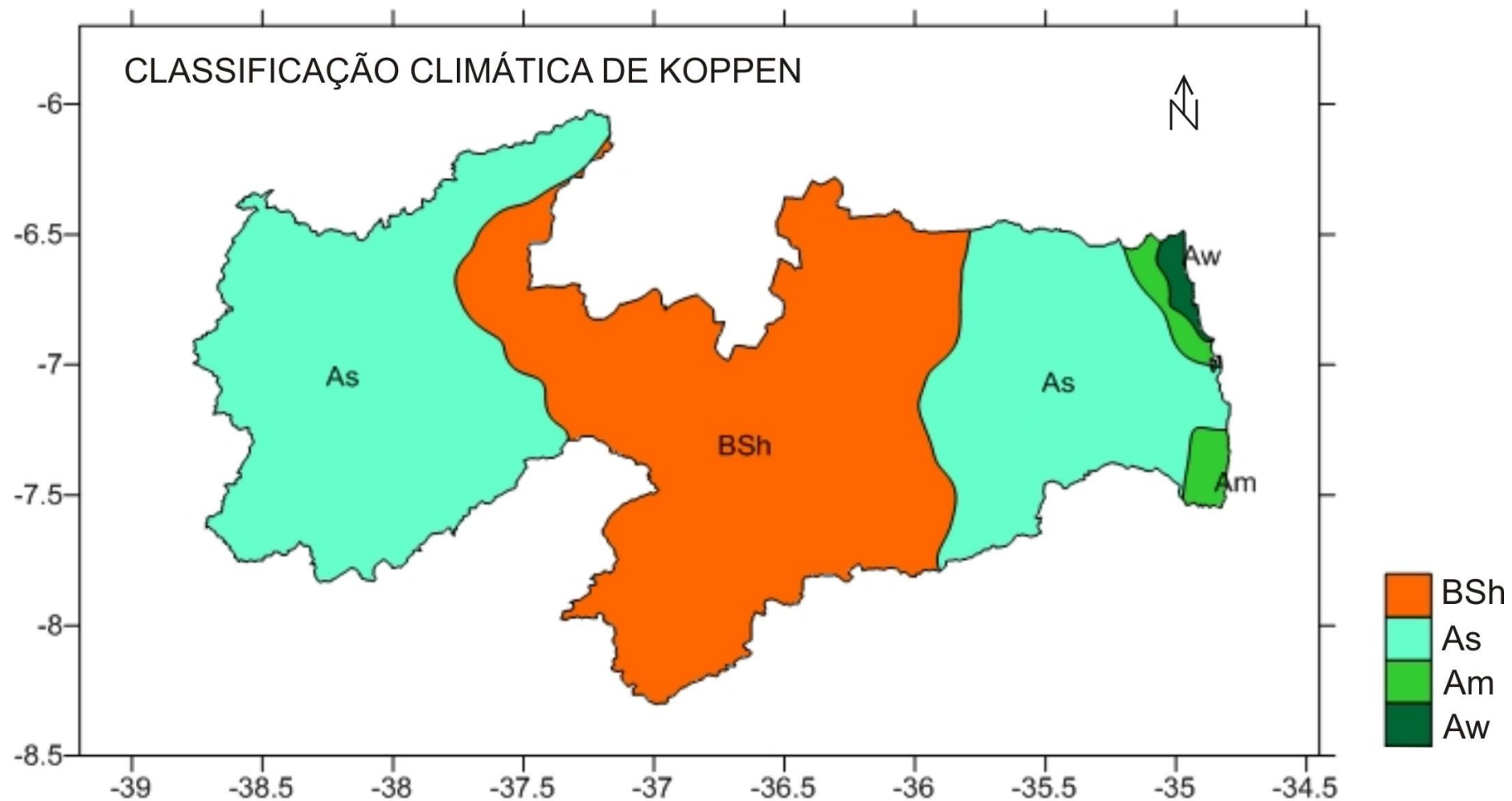
Figura 35. Classificação climática de Köppen.
