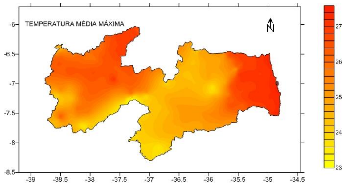
Figura 8. Temperatura média máxima (°C).
