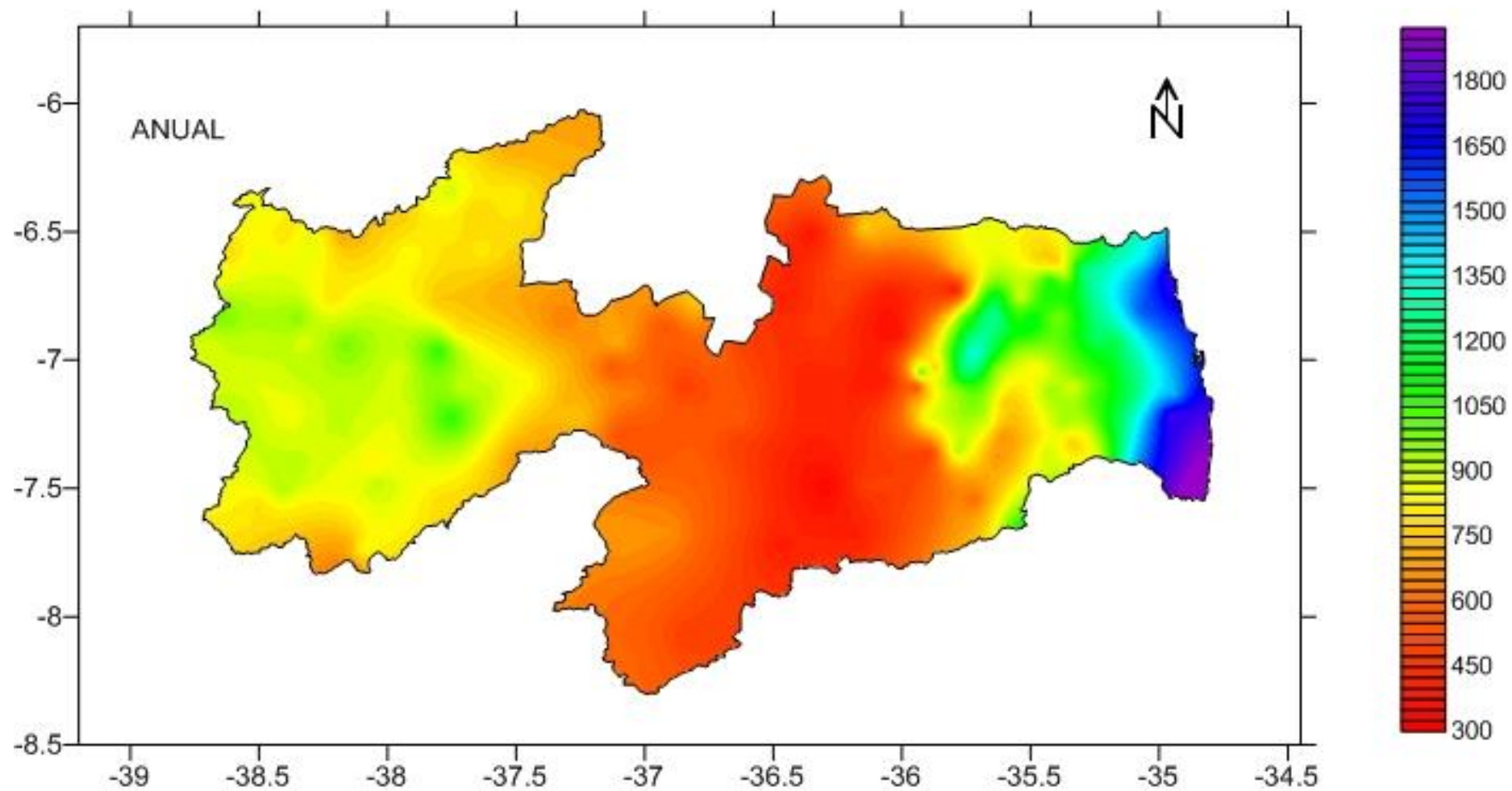
Figura 11. Pluviosidade anual média (mm).
