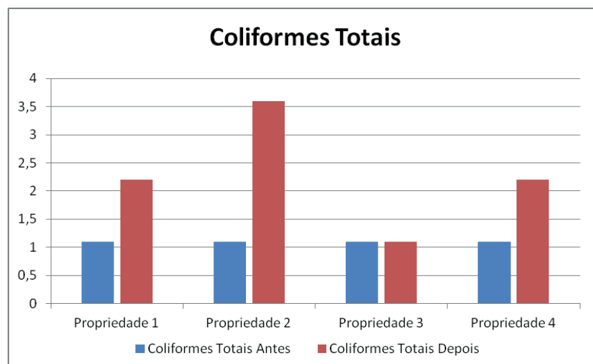
Figura 12: Resultados Coliformes Totais antes e após a recuperação da nascente Fonte: Os autores, 2016
