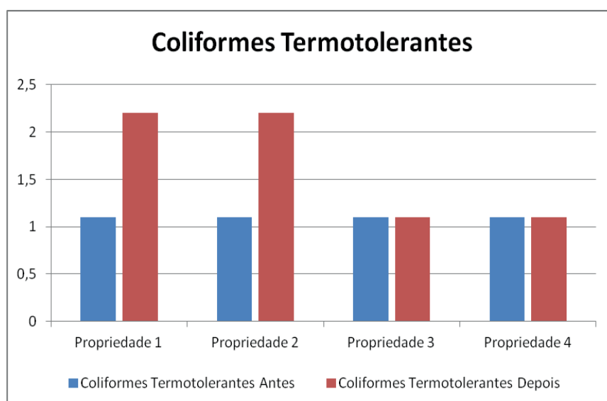
Figura 13: Resultados Coliformes Termotolerantes antes e após a recuperação da nascente Fonte: Os autores, 2016
