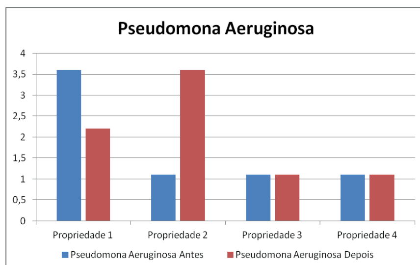
Figura 14: Resultado Pseudomona Aeruginosa antes e após a recuperação da nascente Fonte: Os autores, 2016
