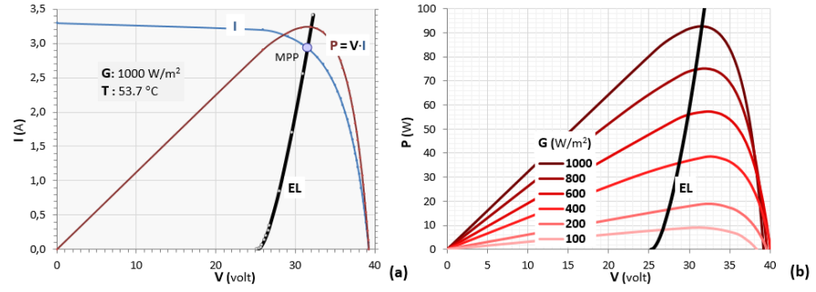
Fig. 3. Acoplamiento FV-EL al MPP ( G_{\max} ) (a) y para otros niveles de radiación (b)
