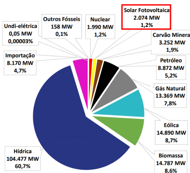
Figura 4: Matriz elétrica brasileira – potência em MW (SAUAIA, 2019).
