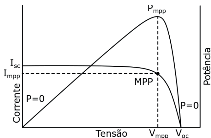
Figura 3. Curva corrente por tensão de um módulo fotovoltaico [5].
