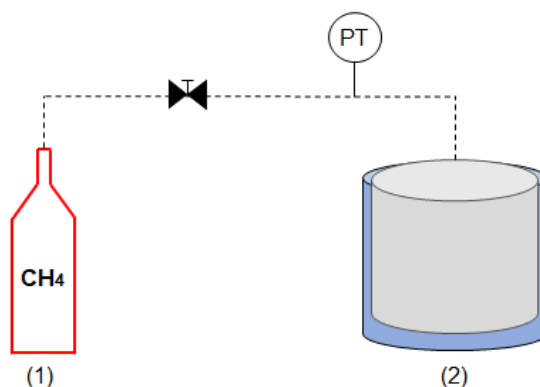
Figura 7 - Esquema simplificado de produção de hidrato em câmara de alta pressão (adaptado de Li et al , 2012): (1) câmara de reação encamisada; (2) cilindro de \text{CH}_4 ; PT - transdutor de pressão.
