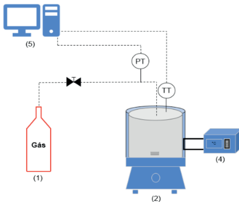
Figura 10 - Fluxograma simplificado do sistema de produção de hidratos de \text{CH}_4 (ABAY, 2011): (1) cilindro de gás; (2) agitador magnético; (3) sistema de refrigeração; (4) computador; PT - transdutor de pressão; TT - sensor de temperatura.
