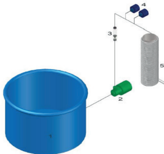
Figura 4 – Circuito hidráulico para floculação do lodo por FTH: I: (1) tanque de efluente; (2) bomba de alimentação; (3) rotâmetro; (4) bombas dosadoras; (5) FTH.
