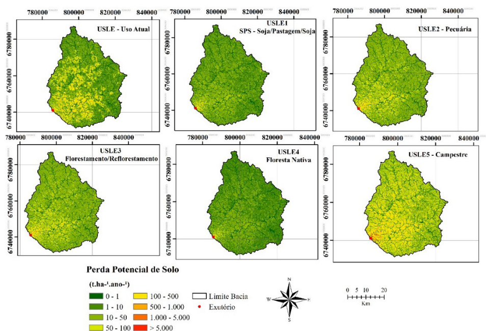
Figura 6 - Mapas de Distribuição de Perda Potencial de Solo, calculada pela equação USLE para diferentes usos do solo nos Cenários USLE, USLE1, USLE2, USLE3, USLE4 e USLE5,
