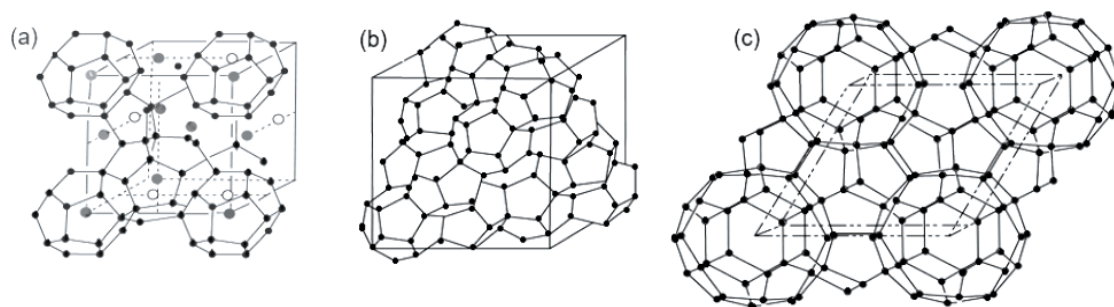
Figura 1 - Estruturas cristalinas formadas nos hidratos de gás (adaptado de SLOAN e KOH, 2008): (a) Estrutura sl (b) Estrutura sII (c) Estrutura sH (adaptado de SLOAN e KOH, 2008).
