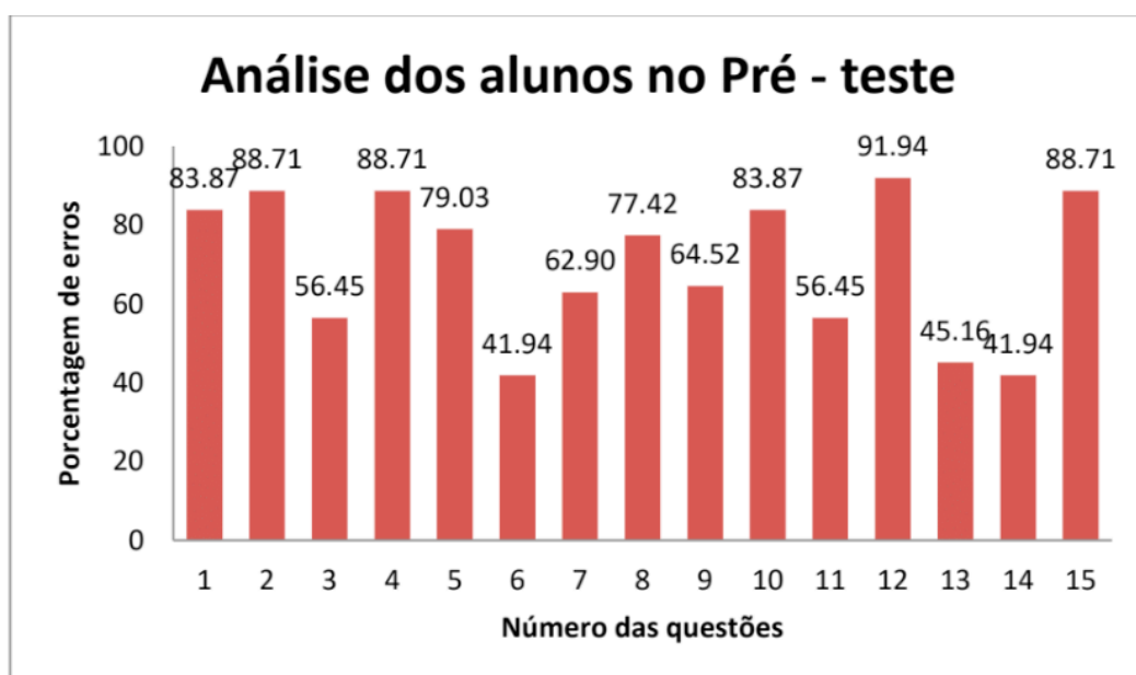
Gráfico 1. Porcentagem de erros dos estudantes no Pré-teste.
