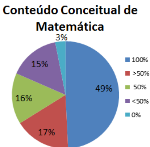
Gráfico 2. Resultado dos estudantes acerca do conhecimento conceitual de matemática – questão 4.
