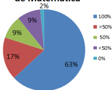
Gráfico 3. Resultado dos estudantes acerca do conteúdo procedimental – questão 5.
