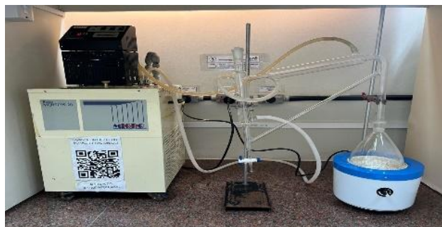
Figura 2. Hidrodestilador Clevenger
