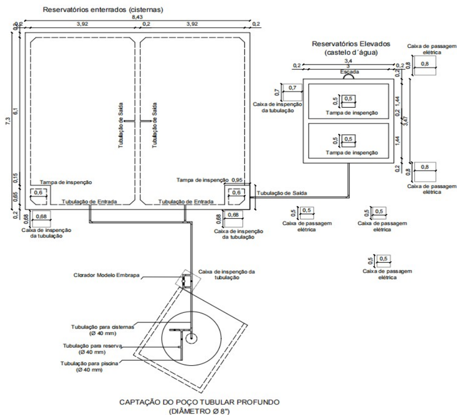
Figura 2 - Planta baixa da SAC com a implantação do clorador.
